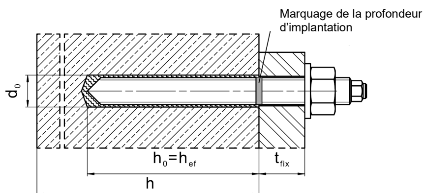
Figure A1 : Tige filetée, HAS-U-... et HIT-V-...
